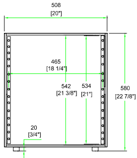
A-A VIEW
