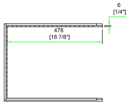
A-A VIEW
