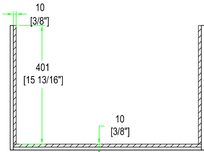
A-A VIEW
