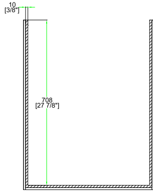
A-A VIEW
